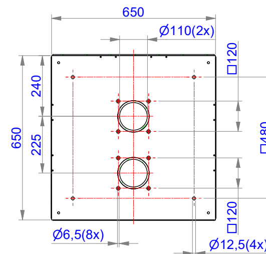
A-A ( 1 : 15 )
